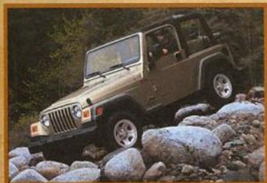
Het indrukwekkende koppel van de 6-in-lijn Power Tech motor helpt de Sport bij steile afdalingen, met "compression braking" oftewel afremmen op de motor.
